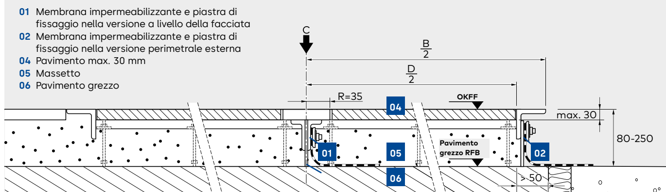
Esecuzione con anello a pavimento e tenuta a livello della facciata con base di raccolta opzionale
