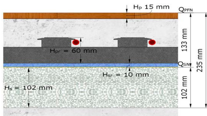
Fig. 9 – Quote considerando lo spessore del massetto nominale o di progetto
