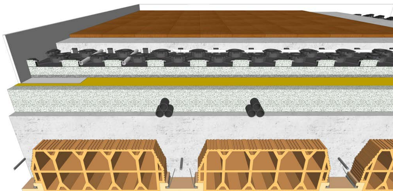
Fig. G.3: Esempio di massetto radiante ribassato su impianto tradizionale e freno al vapore
