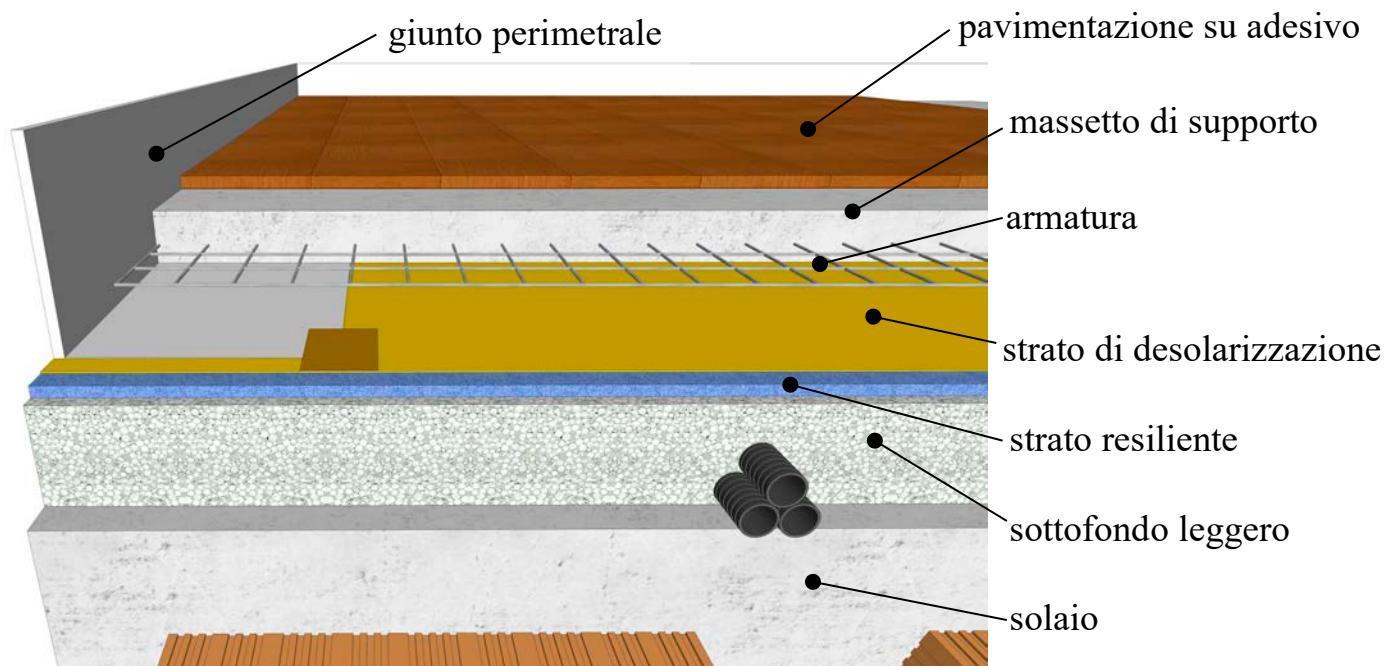
Fig. 2 – Esempio di massetto galleggiante su strato resiliente
