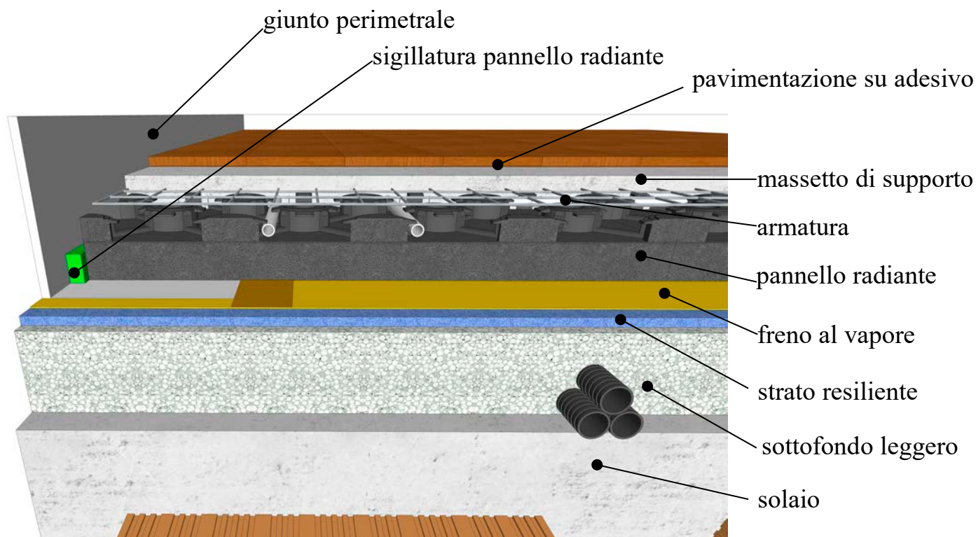
Fig. 3 – Esempio di massetto radiante su strato resiliente
