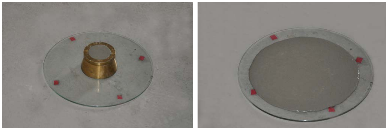
Fig. 5 – Prova di spandimento con cono di Hagerman di un massetto autolivellante
