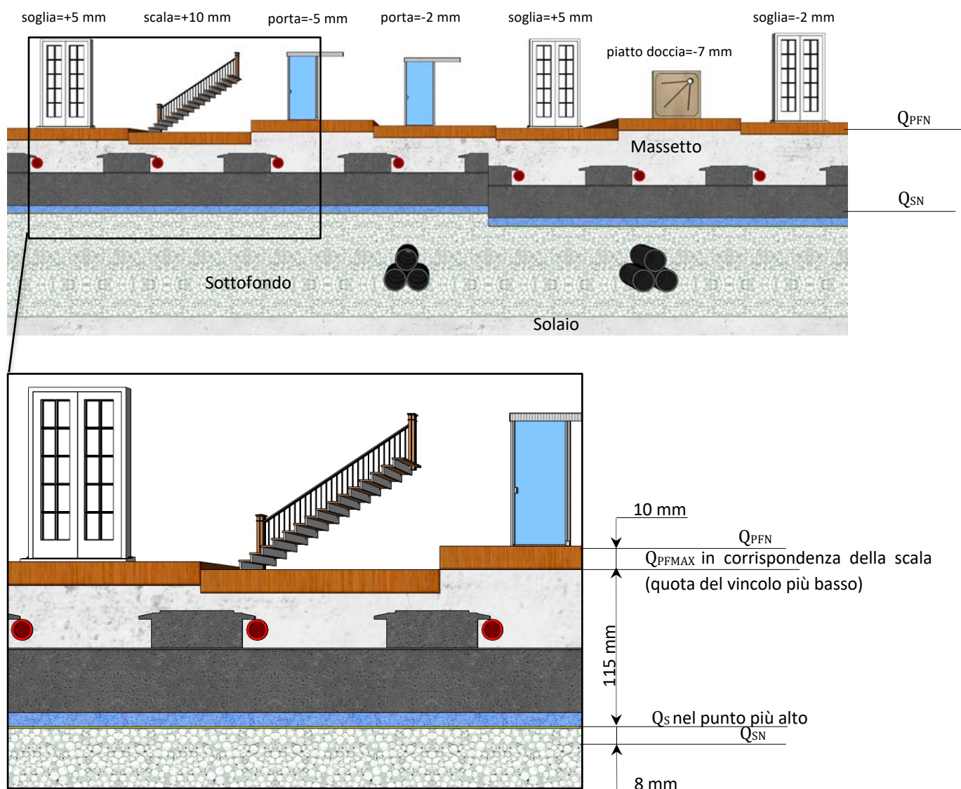
Fig. 8 – Schema che riporta le quote dei vincoli effettive di un appartamento ipotizzato nel Caso A e la tolleranza della quota massima accettabile del sottofondo come da Prospetto 2
