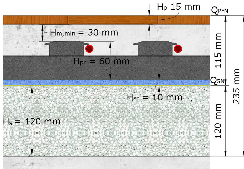
Fig. 7 – Quote considerando lo spessore minimo del massetto
