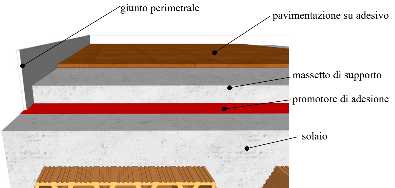
Fig. 4 – Due esempi di massetto aderente al sottofondo
