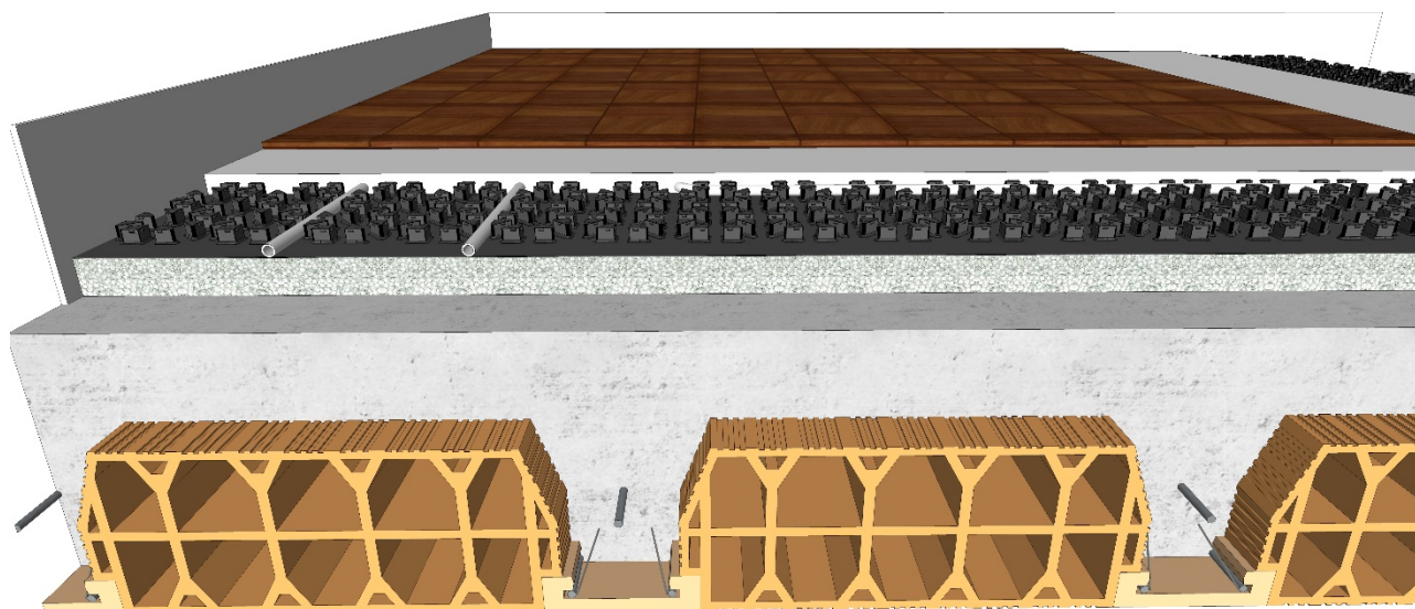
Fig. G.2: Esempio di massetto radiante ribassato a bassa inerzia
