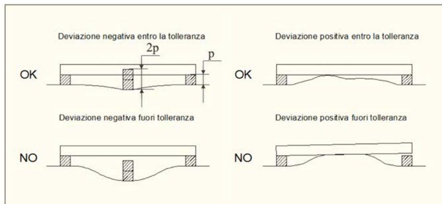
Fig. 13 – Verifica della planarità
