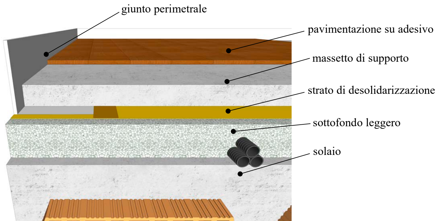
Fig. 1 – Esempio di massetto desolidarizzato su sottofondo leggero
