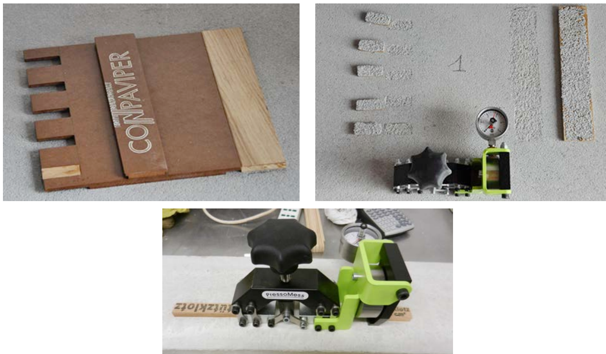
Fig. 14 – Test per la determinazione della resistenza alle sollecitazioni parallele al piano di posa
