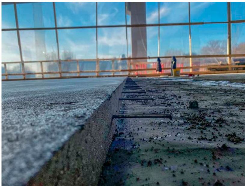
Fig. 20 – Esempio di realizzazione di un giunto di lavorazione
