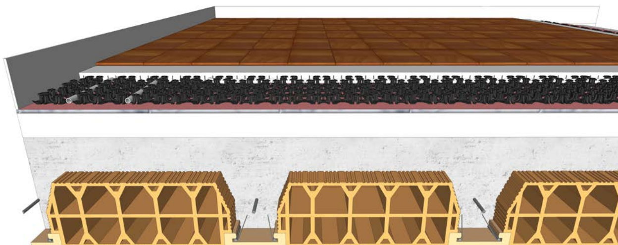
Fig. G.1: Esempio di massetto radiante ribassato in aderenza
