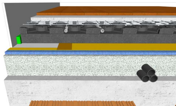
Fig. 23 – Corretto posizionamento del giunto perimetrale nei massetti radianti
