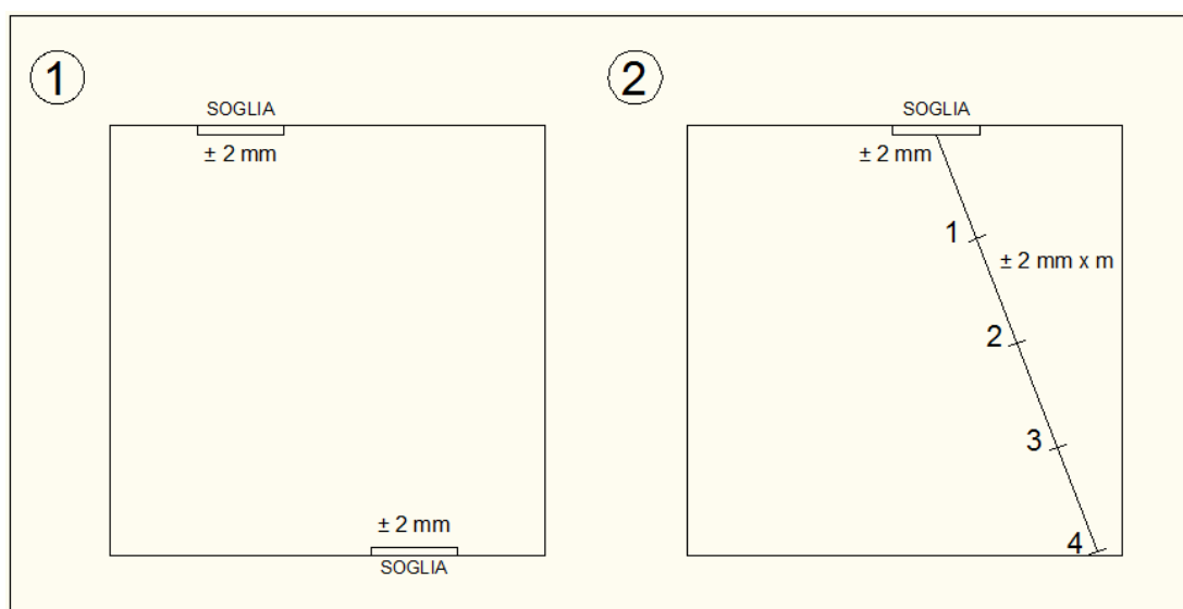
Fig. 12 – Verifica della quota
