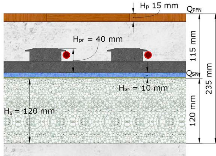
Fig. 11 – Quote considerando lo spessore del massetto nominale o di progetto
