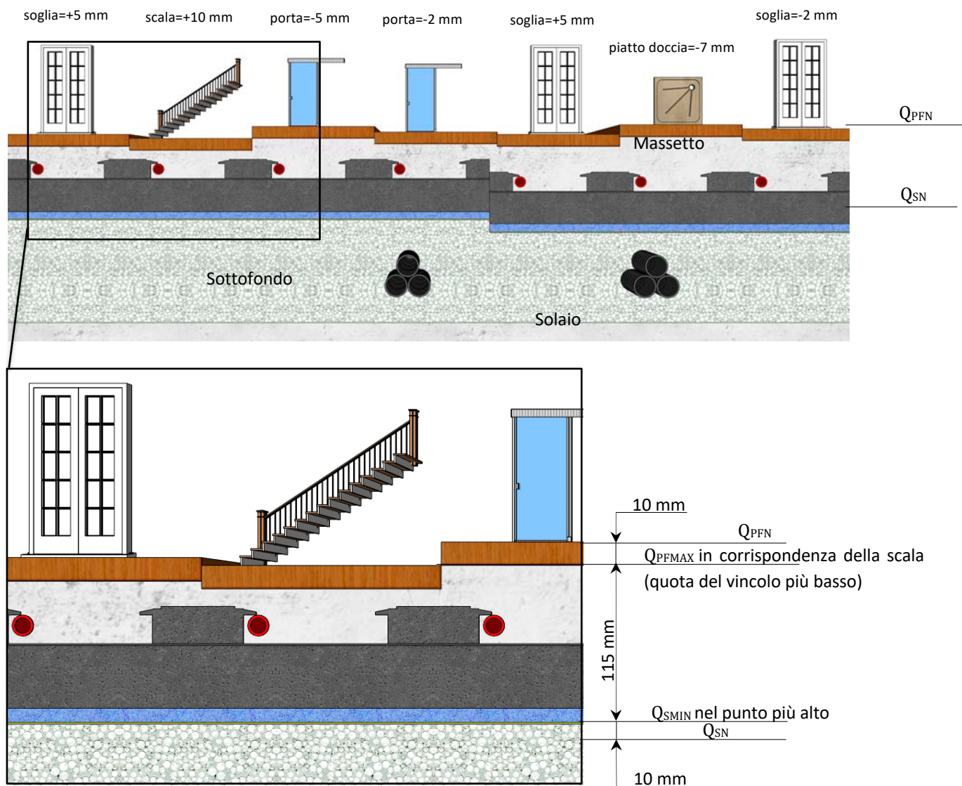
Fig. 10 – Schema che riporta le quote dei vincoli e del sottofondo effettive di un appartamento ipotizzate nel Caso B
