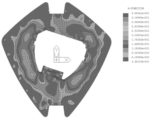
POST-PROCESSING : DENSITA' ARRE ARMATURA
