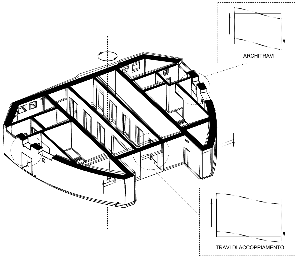
EFFETTI DELLA TORSIONE NEL NUCLEO
