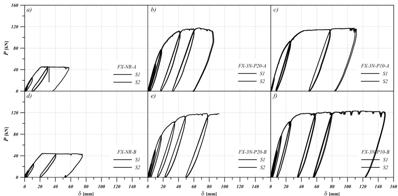
Figura 4 – Curve P- \delta per le travi della tipologia FX
